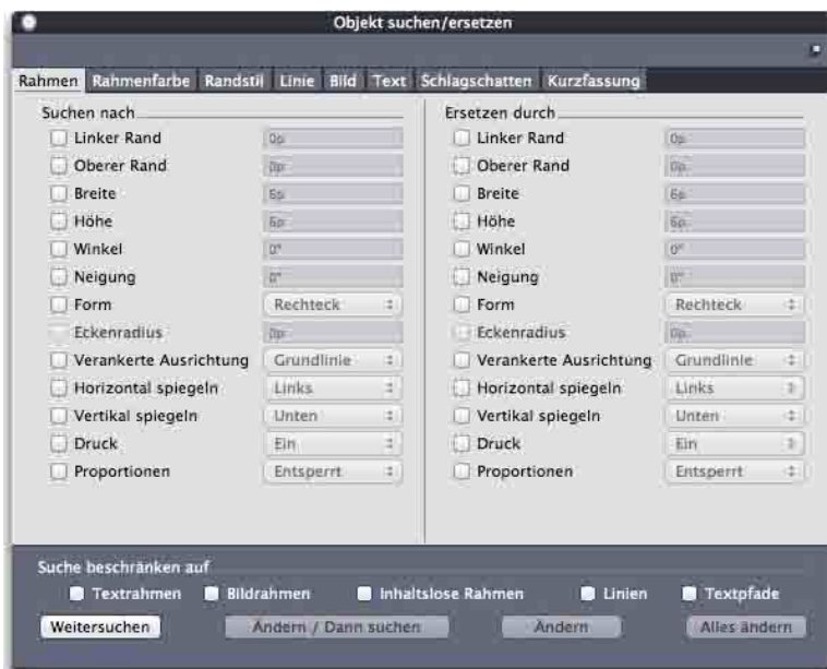
Palette Rechercher/Remplacer
