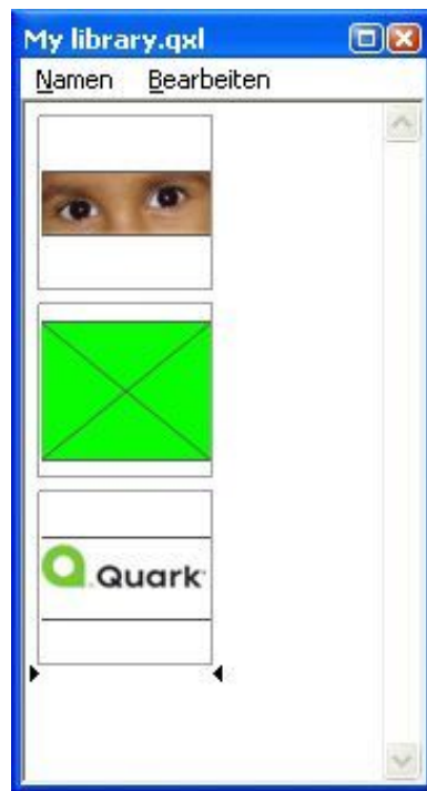
Palette Bibliothèque
